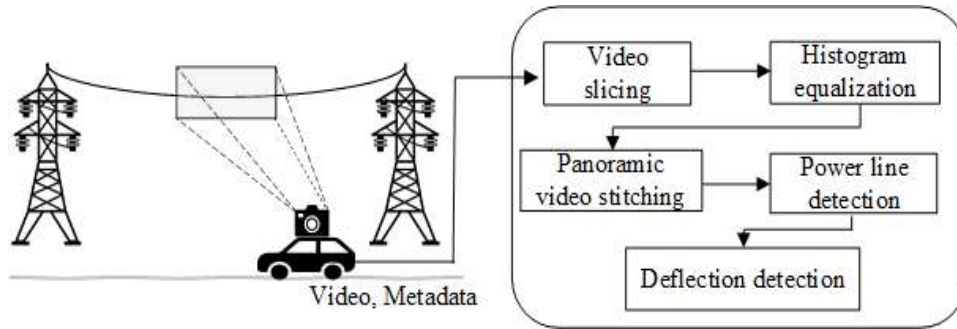
그림 1. 제안하는 딥러닝과 파노라마 영상 스티칭을 이용한 송전선 늘어짐 모니터링 시스템 Fig. 1. Proposed power line deflection monitoring system using deep learning and panoramic video stitching
