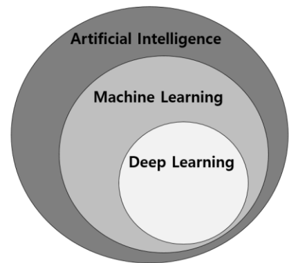
그림 2. 인공지능의 분류
