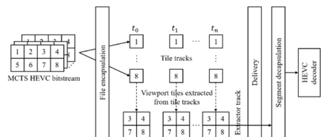
그림 1. 제안하는 다중 타일 추출기 구조도
